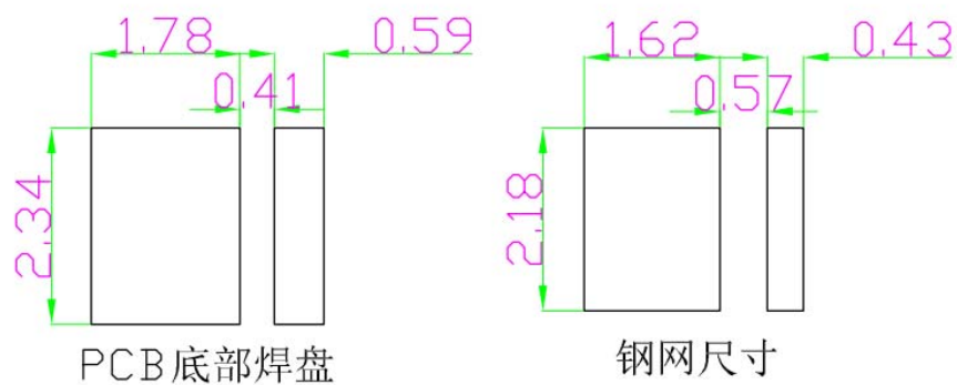
建议焊盘图
