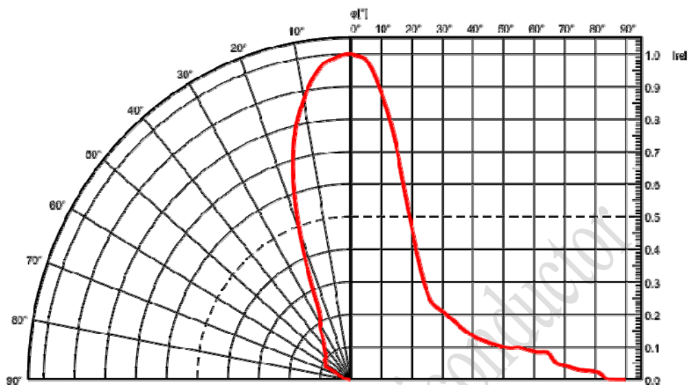
水平方向出光视场角 2\theta_{1/5} 60^\circ HFOV 2\theta_{1/5} 60^\circ
