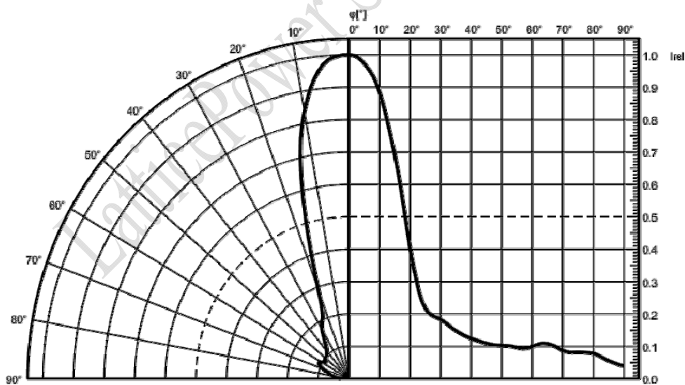
垂直方向出光视场角 2\theta_{1/5} 50^\circ VFOV 2\theta_{1/5} 50^\circ
